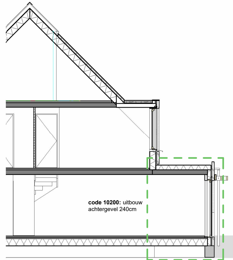
doorsnede
