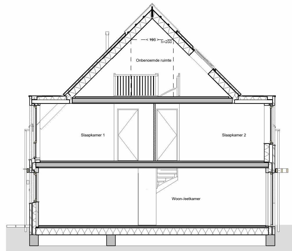
doorsnede
