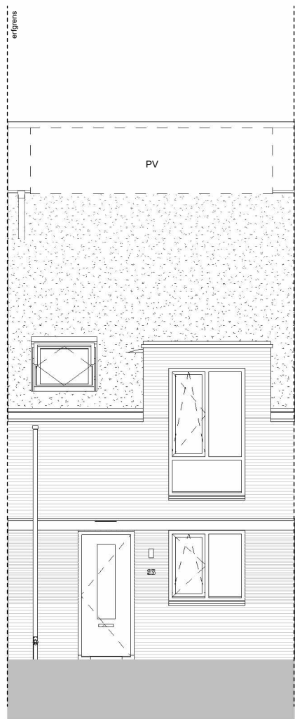
voorgevel
